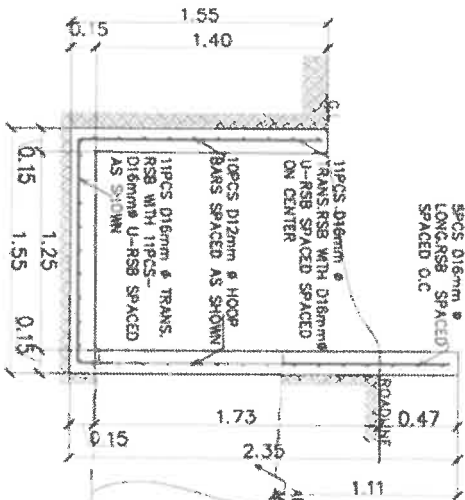
SECTION THRU A-A SCALE 1:30
