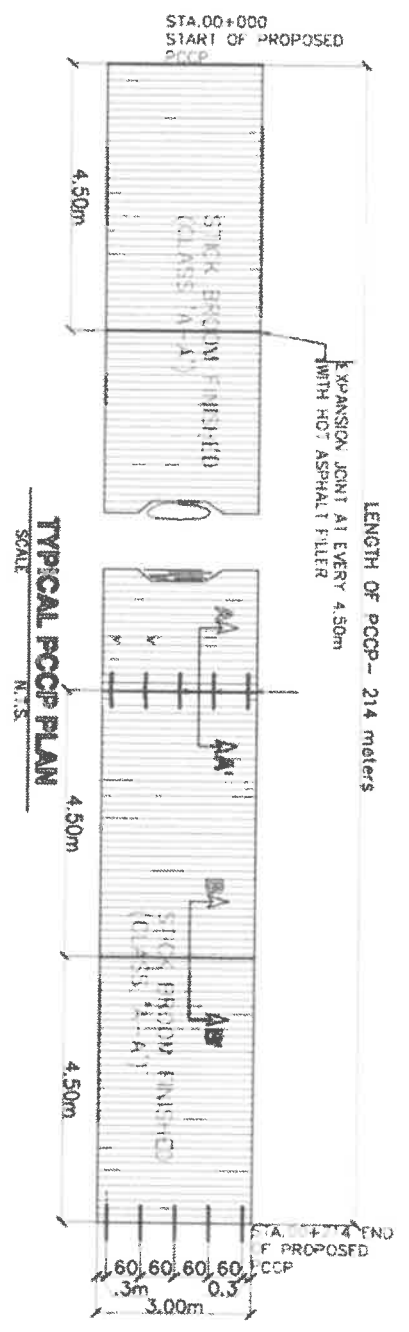
GENERAL PLAN SCALE N.T.S.
