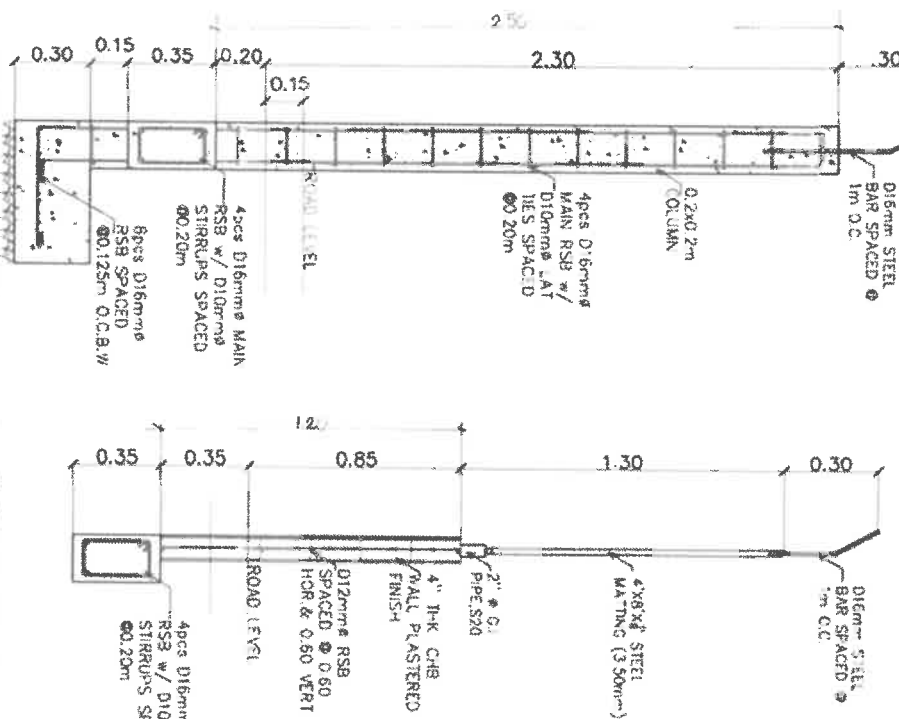
TYP. SECTION THRU A-A SCALE 1:20
